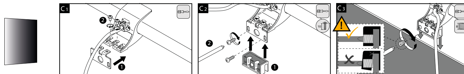
C Assembly in glass / Montaggio di vetro / Montaje en cristal / Montage en verre / Montagem de vidro / Montaż w szkle / Montage in Glas
