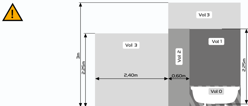
PROTECTION VOLUMES / ZONE DI PROTEZIONE / VOLÚMENES DE PROTECCIÓN / VOLUMES DE PROTECTION / VOLUMES DE PROTECÇÃO / OPRAWY / SCHUTZBEREICHE
