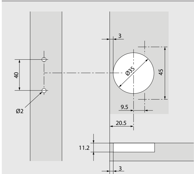
Padrão de Furação
