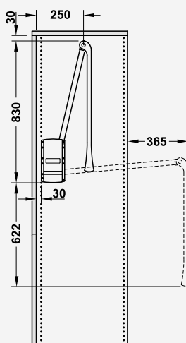
Instalação na fileira traseira de furos em série
