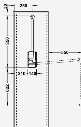
Instalação no centro do painel lateral do guarda-roupa
