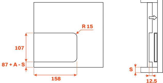
Usinagem da lateral sobreposta
