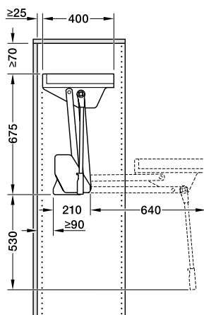
Dimensões de construção prateleira de madeira
