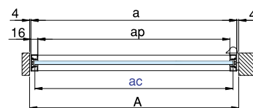
Perfil horizontal
