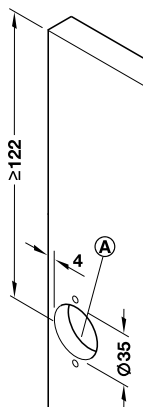
A Profundidade de furação de dobradiça invisível
